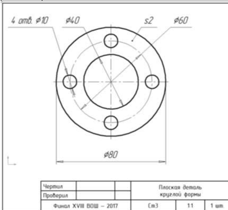
Рис. 1. Образец чертежа плоской детали круглой формы
